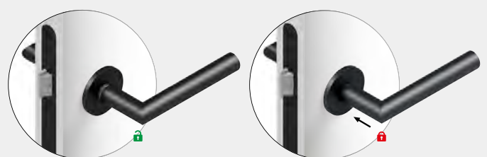
Axialdruck verriegelt | Axialzug entriegelt
