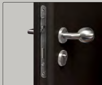
PZ-Schloss, Klasse 5 mit verstärktem Stulp
