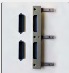
WE-Schließblech mit Stahllaschen
